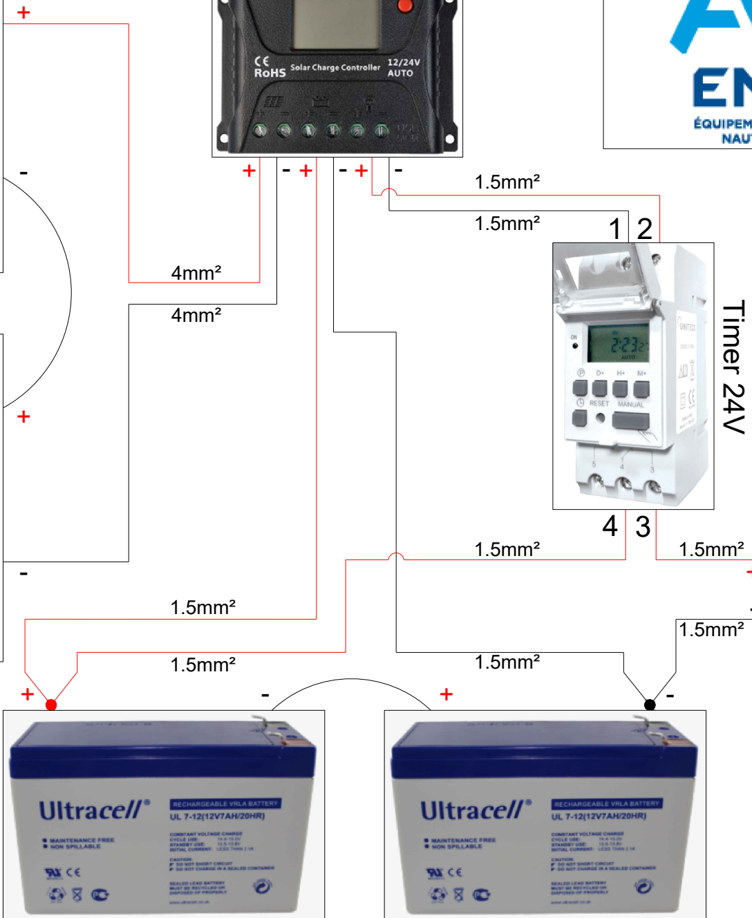
Batterie 12V
